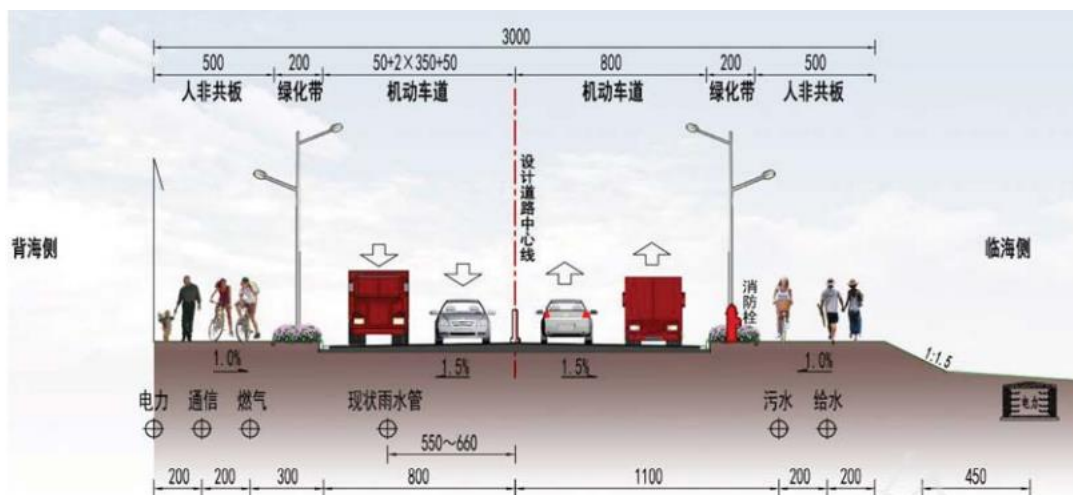
图 2.3.2-1 西大堤（海滨大道～黄石嘴段）（K0+000~K0+406.5）标准横断面图
