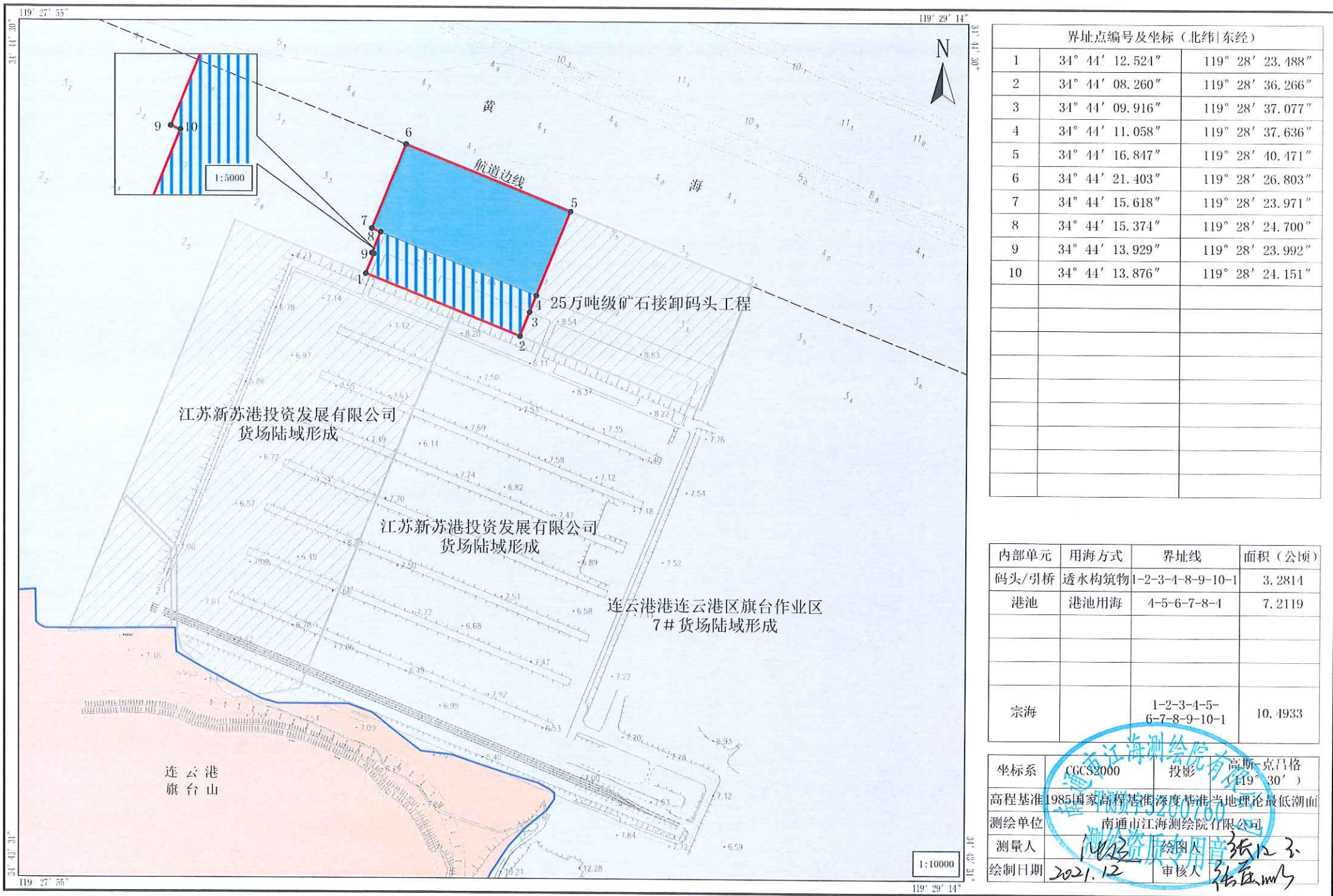
连云港港旗台作业区10万吨级通用散货泊位工程项目宗海界址图
